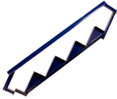
Forma de Escada Jacaré (6 degraus)
